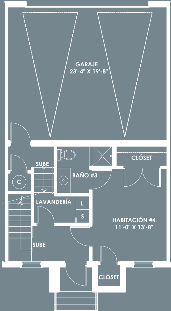
PRIMERA PLANTA
