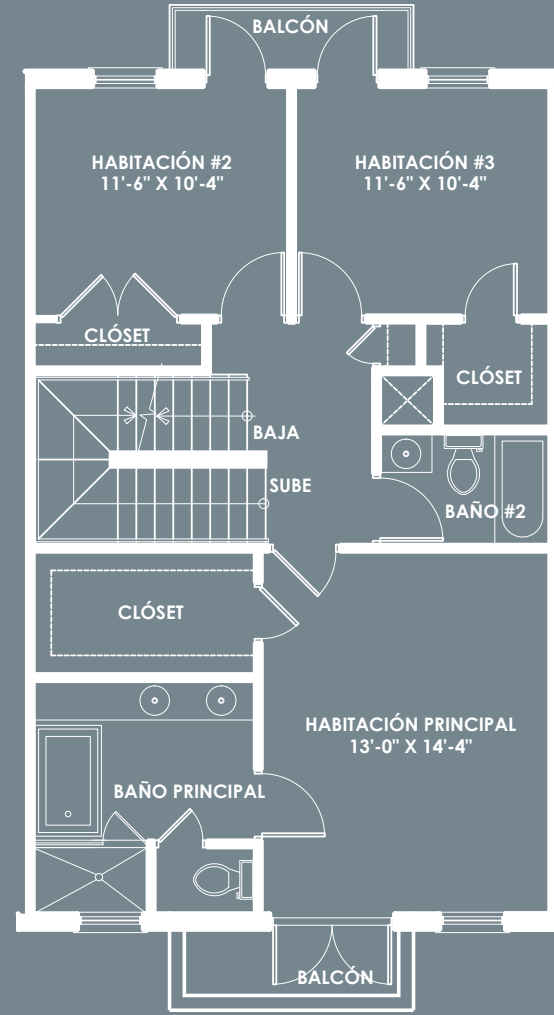
TERCERA PLANTA
